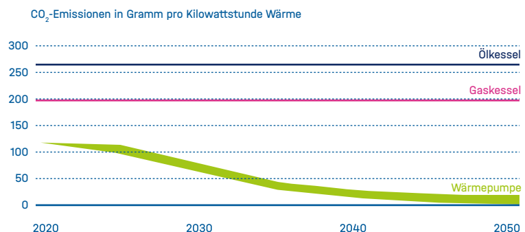
Grafik: Entwicklung des Emissionsfaktors von Öl- und Gaskesseln im Vergleich zu Wärmepumpen. Der Emissionsfaktor zeigt, wie viel Treibhausgasemissionen je kWh bereitgestellter Wärme entstehen. © Wüstenrot Stiftung/Forschungsstelle für Energiewirtschaft e.V.
