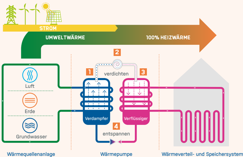
Grafik: Funktionsprinzip Wärmepumpe © Bundesverband Wärmepumpe (BWP) e.V.
