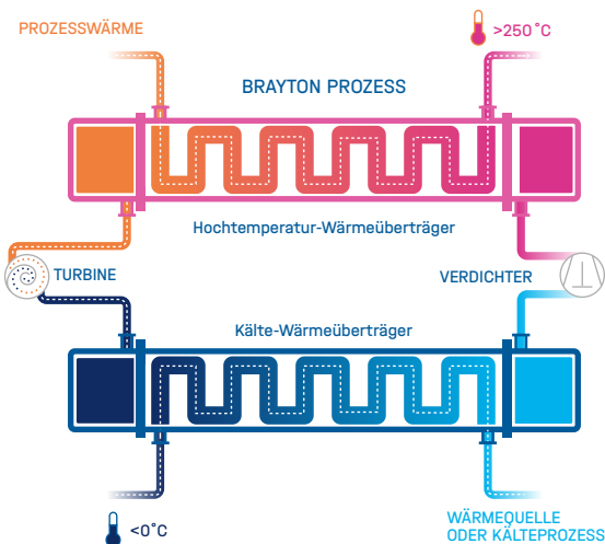
Grafik: Die Funktionsweise der CoBra-Pilotanlage © Das DLR-Institut für CO 2 -arme Industrieprozesse
