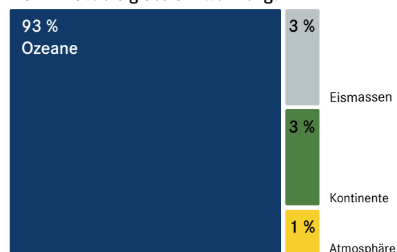
Wohin fließt die globale Erwärmung?
